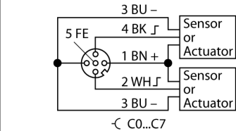
Napájecí konektor 7/8"
