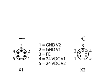
Napájecí konektor 7/8"
